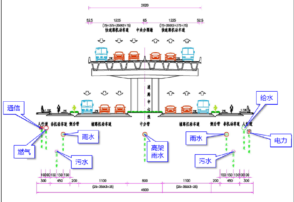
图 2.5-6 本项目管线综合布置图
