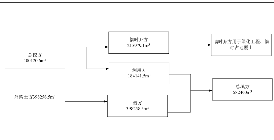
图 2.5-7 本项目土石方平衡表
