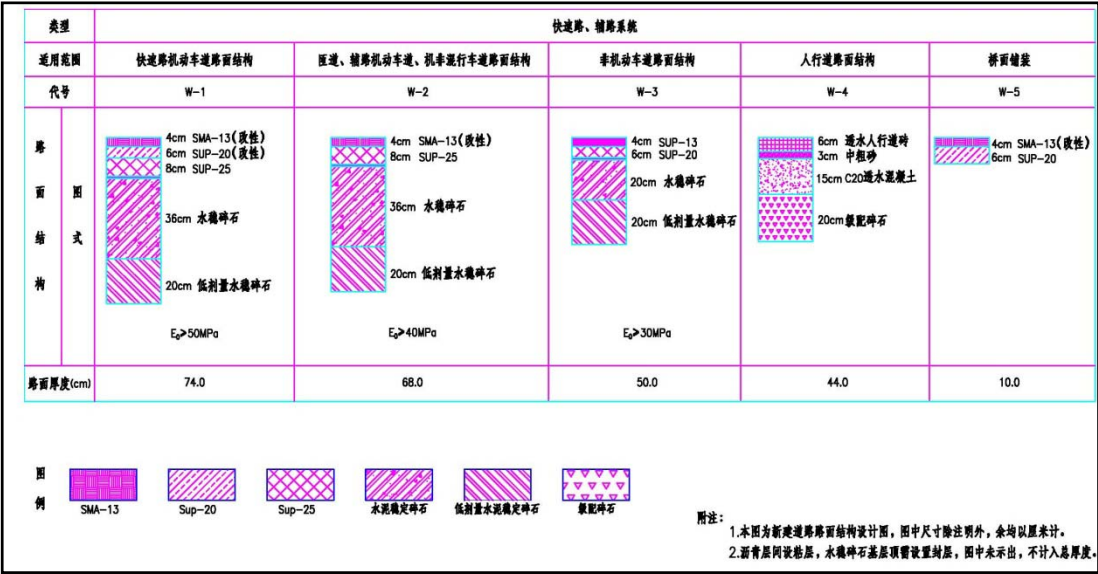
图 2.5-2 项目路面结构形式一览表
