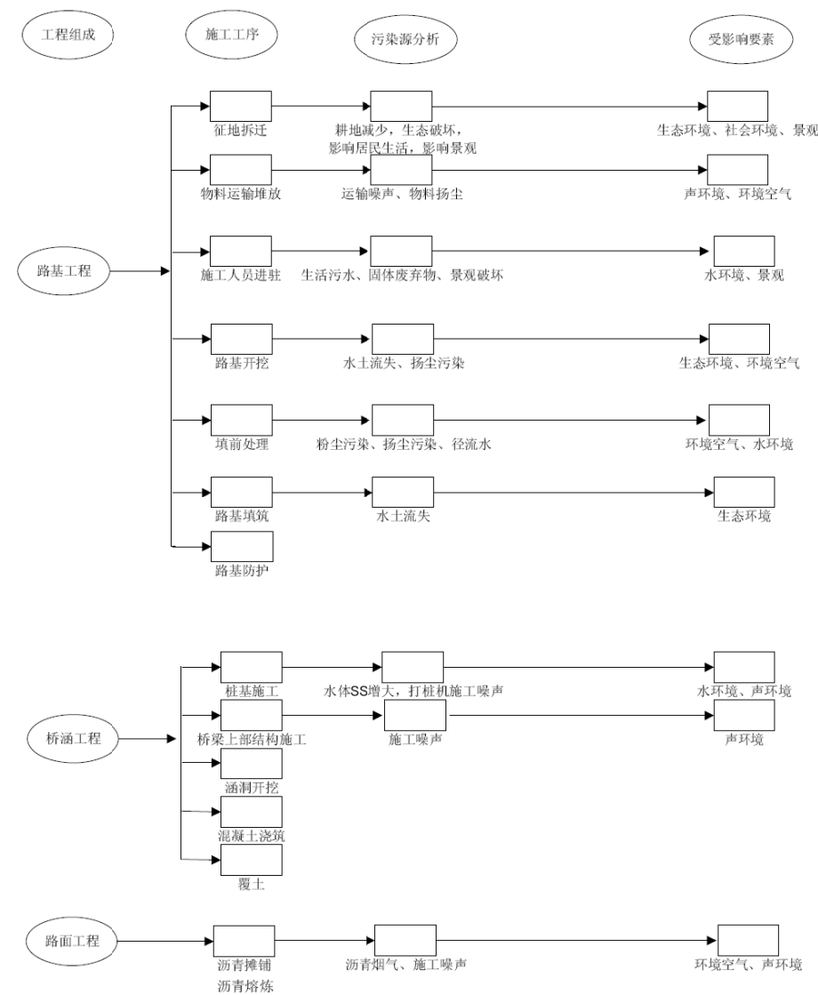
图 6.1-1 施工期污染源分析
