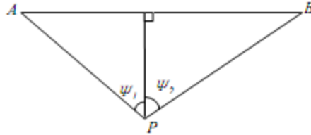
图 8.1-1 有限路段的修正函数，A-B 为路段，P 为预测点
